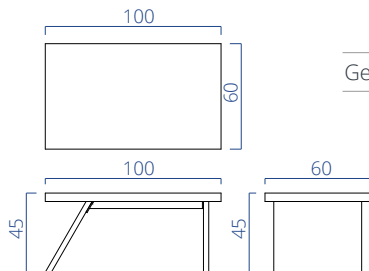
A05DM100 Damla Sehpa/Coffee Table
