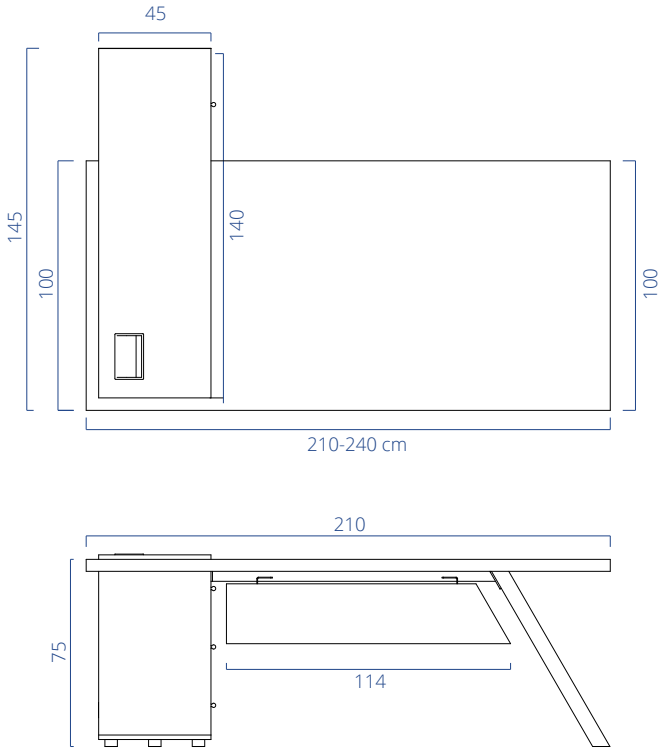
A01DM211 Damla 210 cm Sol Etajerli Masa/Right Side Table
